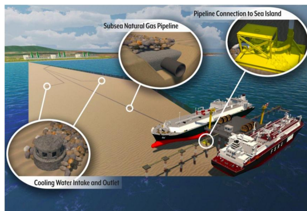
Thiết kế hệ thống neo và hệ thống ống chìm cung cấp khí cho nhà máy điện từ FSRU
