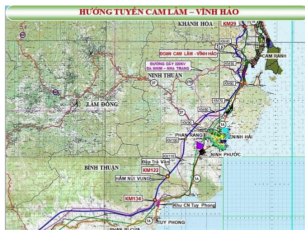
Sơ đồ đoạn cao tốc Cam Lâm - Vĩnh Hảo (đường màu xanh) do đơn vị tư vấn đề xuất
