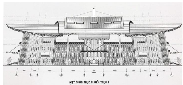
Bản thiết kế mặt đứng công trình nhà hát và triển lãm. (Ảnh tư liệu)
